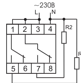
Рис.1 Рекомендуемая схема подключения таймера PCZ-522 и нагрузки к сети 230В.
